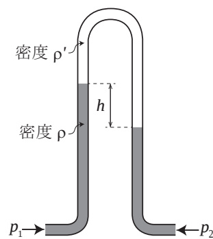
図 3: U 字管マノメータ
