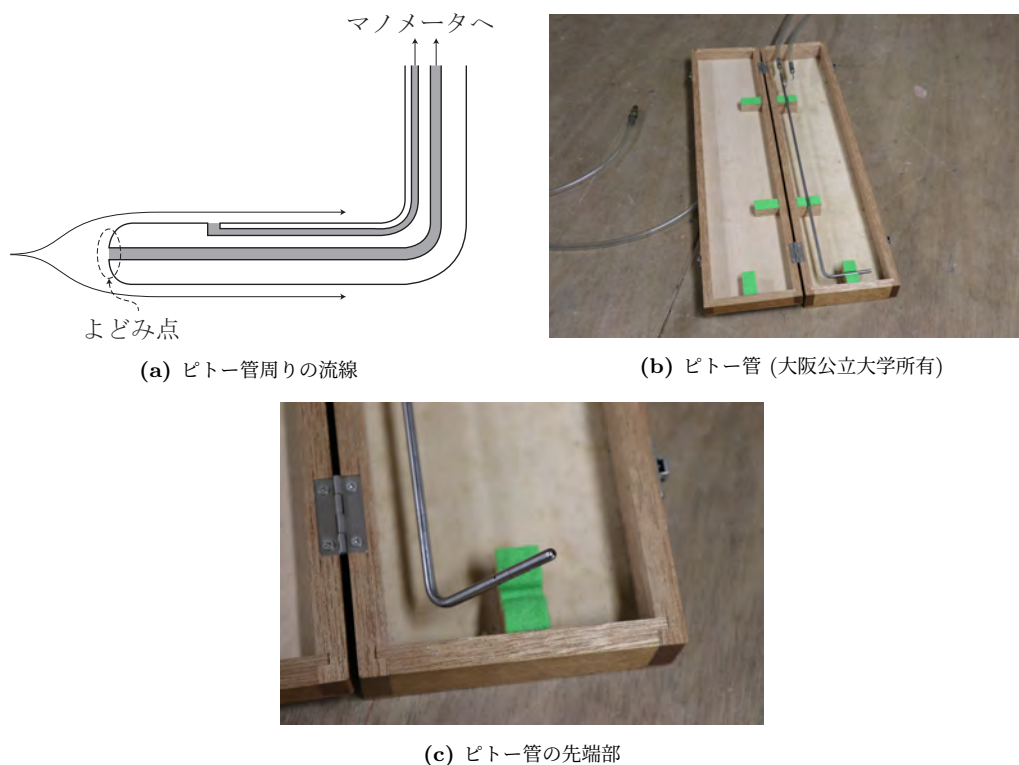
図4: ピトー管 (Pitot tube)
